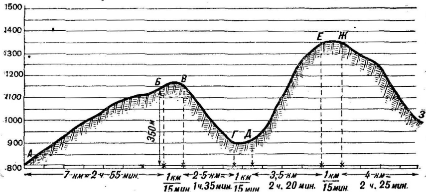
Схема 3. Профиль пути для расчета времени на марш.
